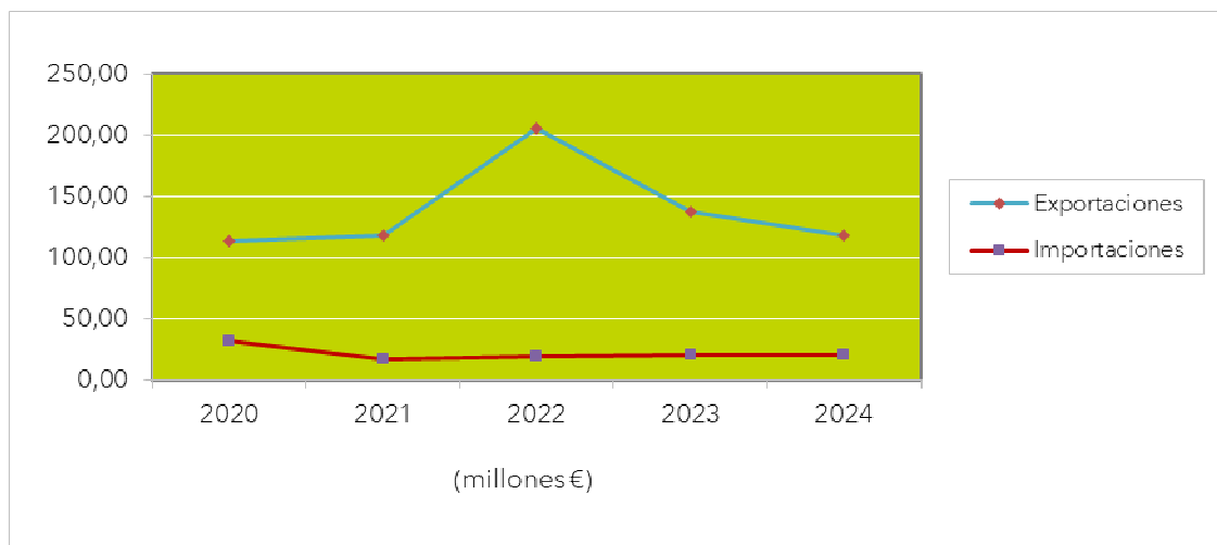
Gráfico 2. Evolución exportaciones Murcia-Japón. 2020-2024
